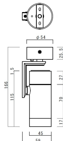
フランジタイプ
