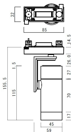
ダブルフック (ダクトレール用)
