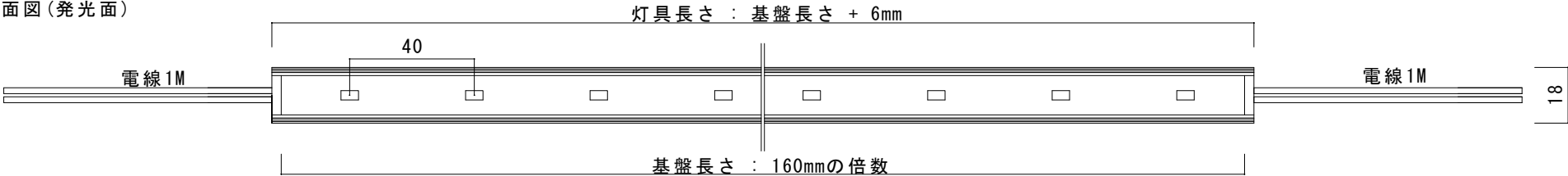
正面図(発光面)
