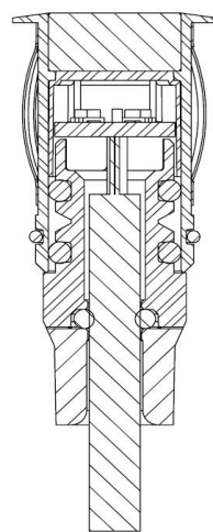
SECCIÓN A-A
