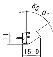
ブラケット金物装着時
